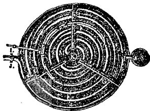
Фиг. 5 и 6. Аппаратъ Фуше для нагреванія сыраца глухимъ паромъ.
