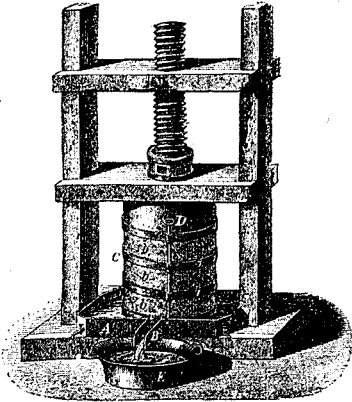
Фиг. 2. Прессъ для выжимки сала изъ шквары
