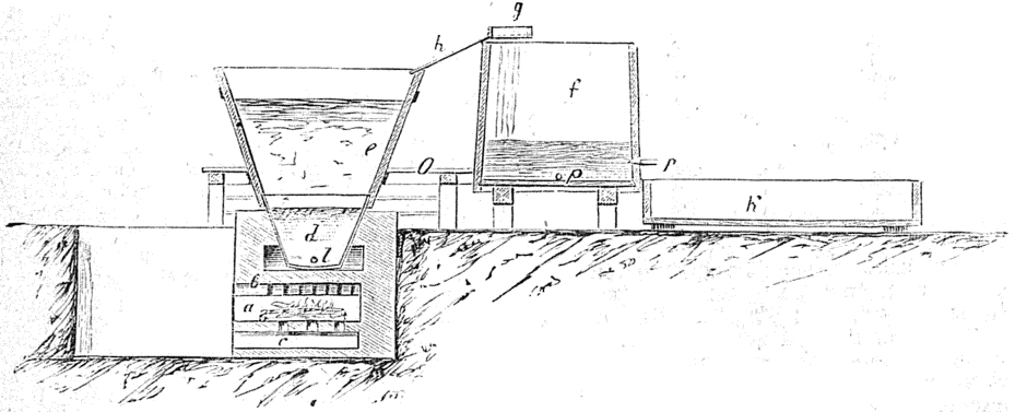
Фиг. 1. Схема салотопления на небольших русских салотопных заводах. a —топка подъ котломъ; c —зольникъ; d —металлическая часть салотопнаго котла; e —наставка; f —отстойный чанъ; g —сито; h —желобъ, по которому шквара съ сѣта счищается въ котель; k —холодный ларь; l —отверстие для выпуска воды и шквары. p —отверстия для выпуска сала; o —помость
