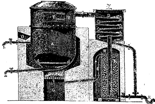
Фиг. 4. Аппаратъ Воля.
