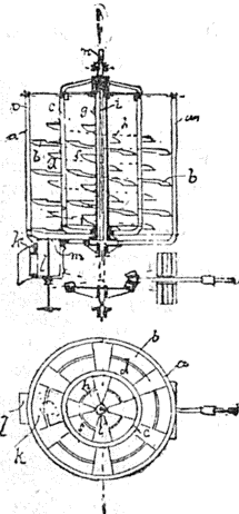
Фиг. 3. Аппаратъ Отто Эйзенверка
